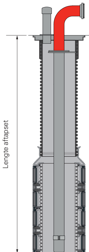
Voorbeeld: QuadroTake 1 met pompschacht
