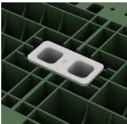
Enkellaagse verbindingsclip
