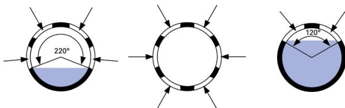
Gedeeltelijk geperforeerde drainagebuis (LP)
